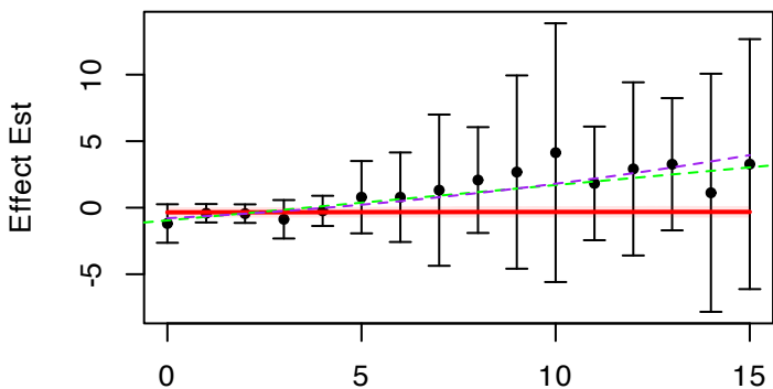
ITGA3: rs199143
