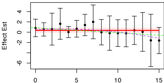
TSPAN9: rs11062517
